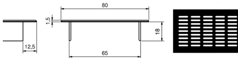
Grille d'aération en aluminium avec hauteur 80 mm
