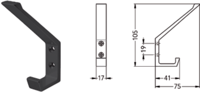
Portemanteau type 138 - avec porte-chapeau
