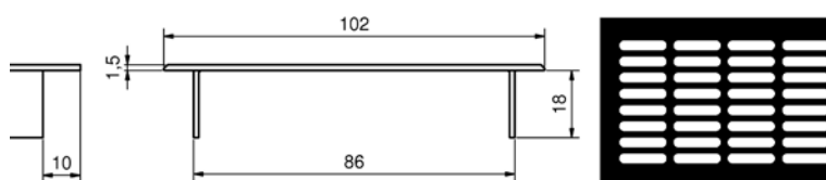
Grilles d'aération en aluminium avec hauteur 102 mm
