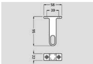
Supports type 1190 et 1192
