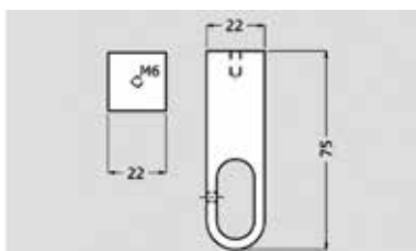
Supports type 1194 et 1196
